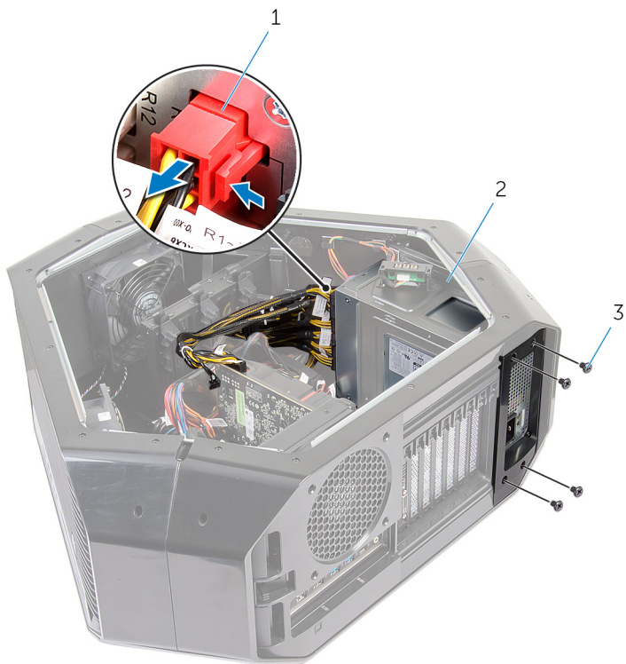
図 47. 電源装置ユニットの取り外し
