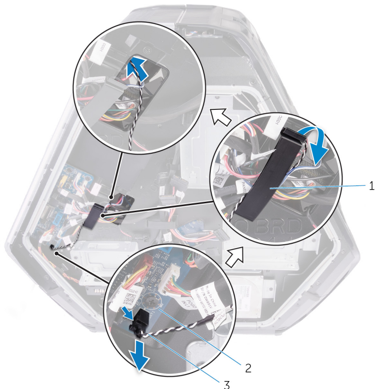
図 64. 背面 I/O アクセシビリティ照明ケーブルの取り外し
