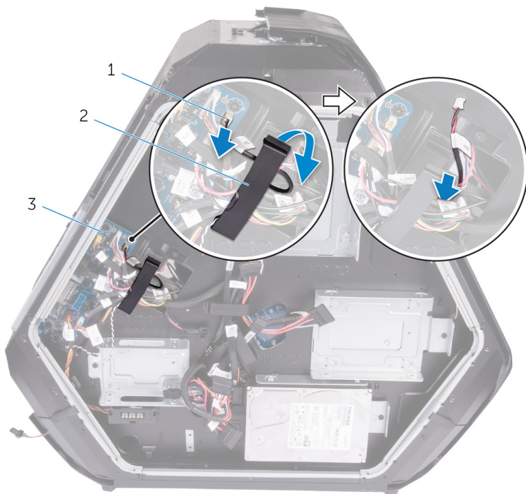
図 61. オプティカルドライブ取り出しボタンボードケーブルの取り外し
