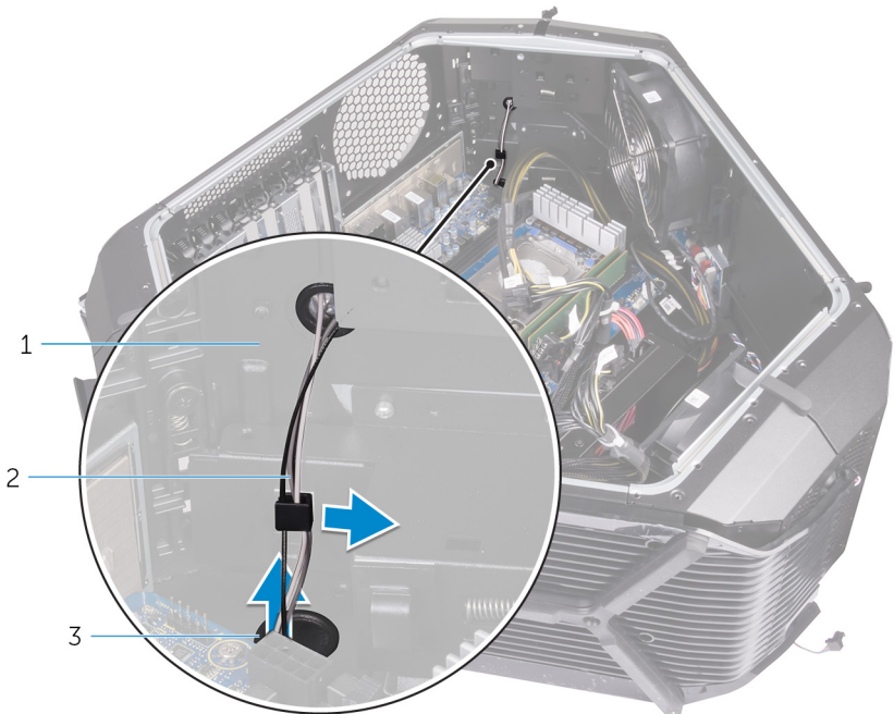
図 80. アンテナケーブルの取り外し
