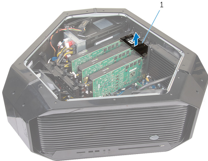
図 27. グラフィックスブリッジの取り外し
