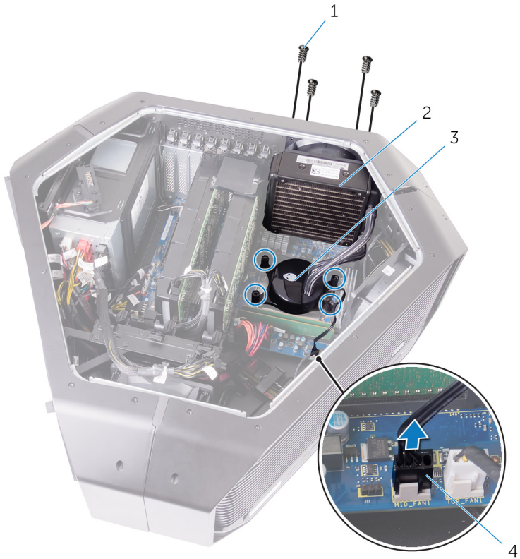
図 45. プロセッサ液体冷却アセンブリの取り外し
