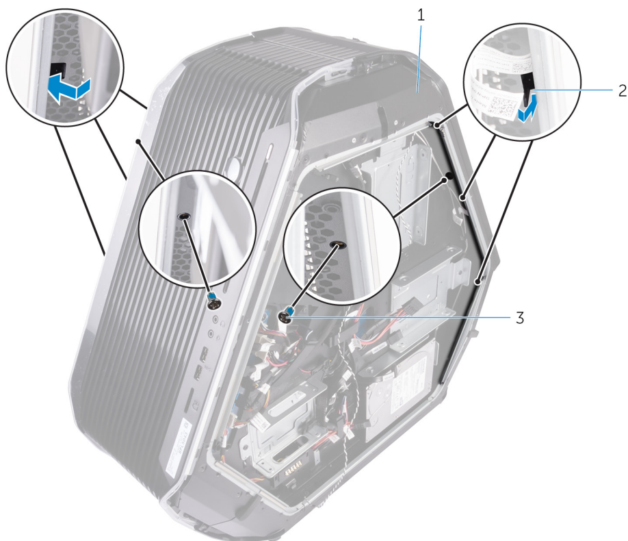
図 68. 背面ベゼルの取り外し
