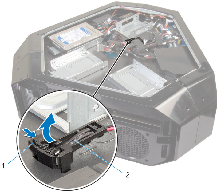
図 23. ドライブベイ熱センサーケーブルの取り外し
